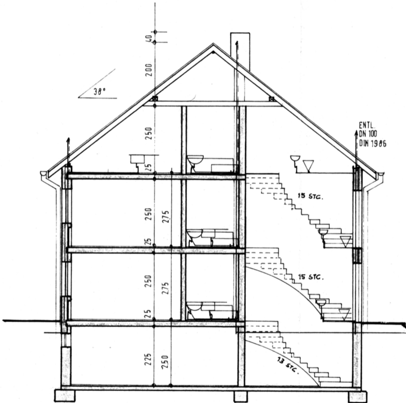
SCHNITT "A-B"
